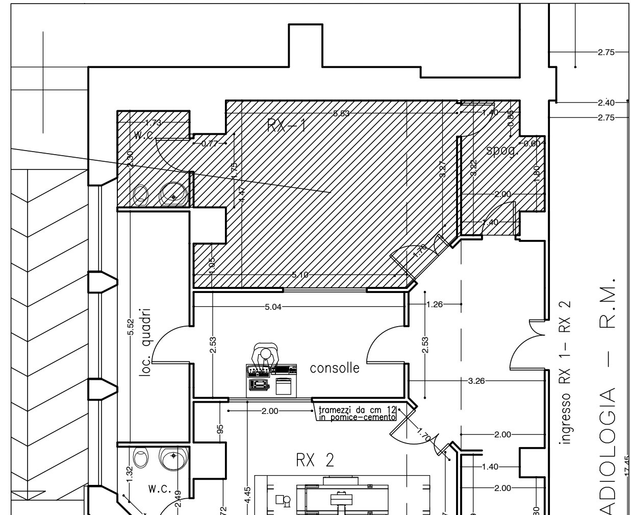
LOTTO 2: LOCALE INDIVIDUATO PER REALIZZAZIONE DI UN SISTEMA RADIOLOGICO TELECOMANDATO DIGITALE DIRETTO MULTIFUNZIONALE DI MQ 36
